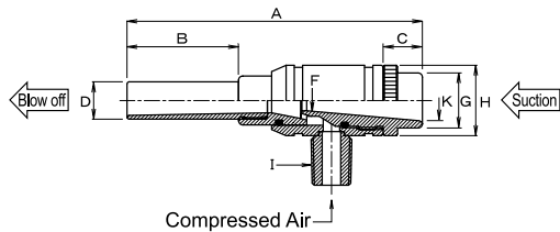
W501-S(G) W501-L(G)
